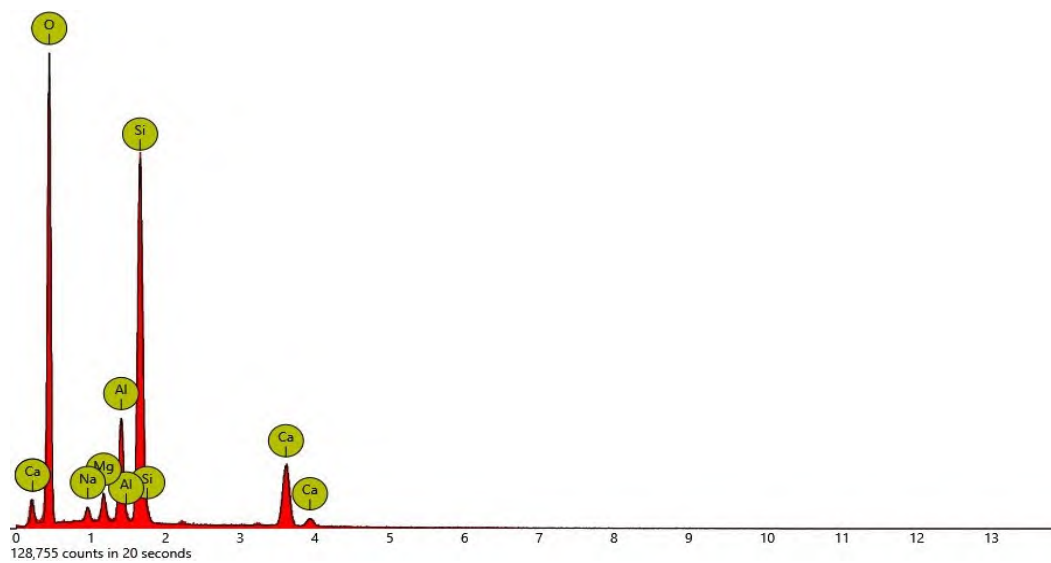
Bild 4: EDX-Spektrum Steinwolle
